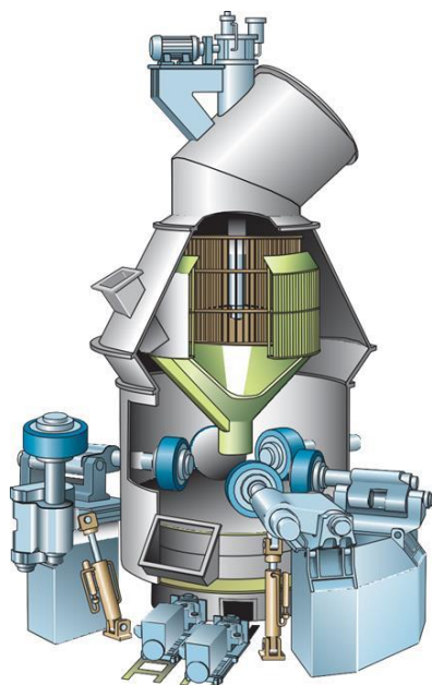
Vertikální mlýn
